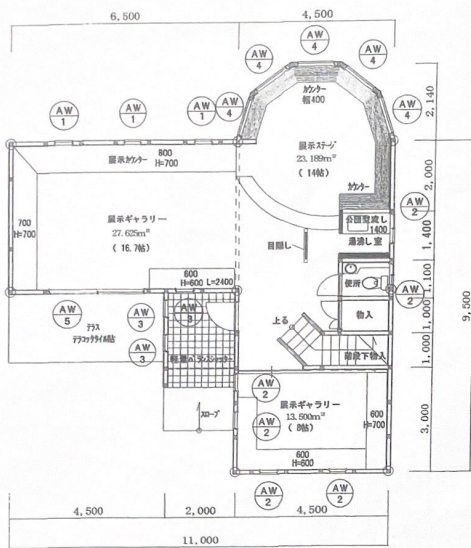
1階平面図 1:100
